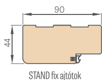
STAND fix ajtótok
