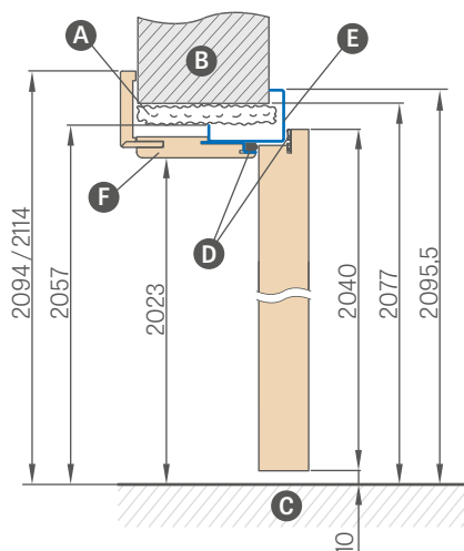
1 elemes ajtótok, 140-260mm tartományban állítható, 20 mm-enként
