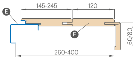
2 elemes ajtótok, 260-400mm tartományban állítható, 20 mm-enként
