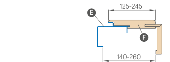
1 elemes ajtótok, 140-260mm tartományban állítható, 20 mm-enként
