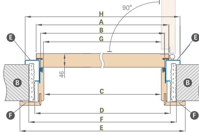
2 elemes ajtótok, 260-400mm tartományban állítható, 20 mm-enként
